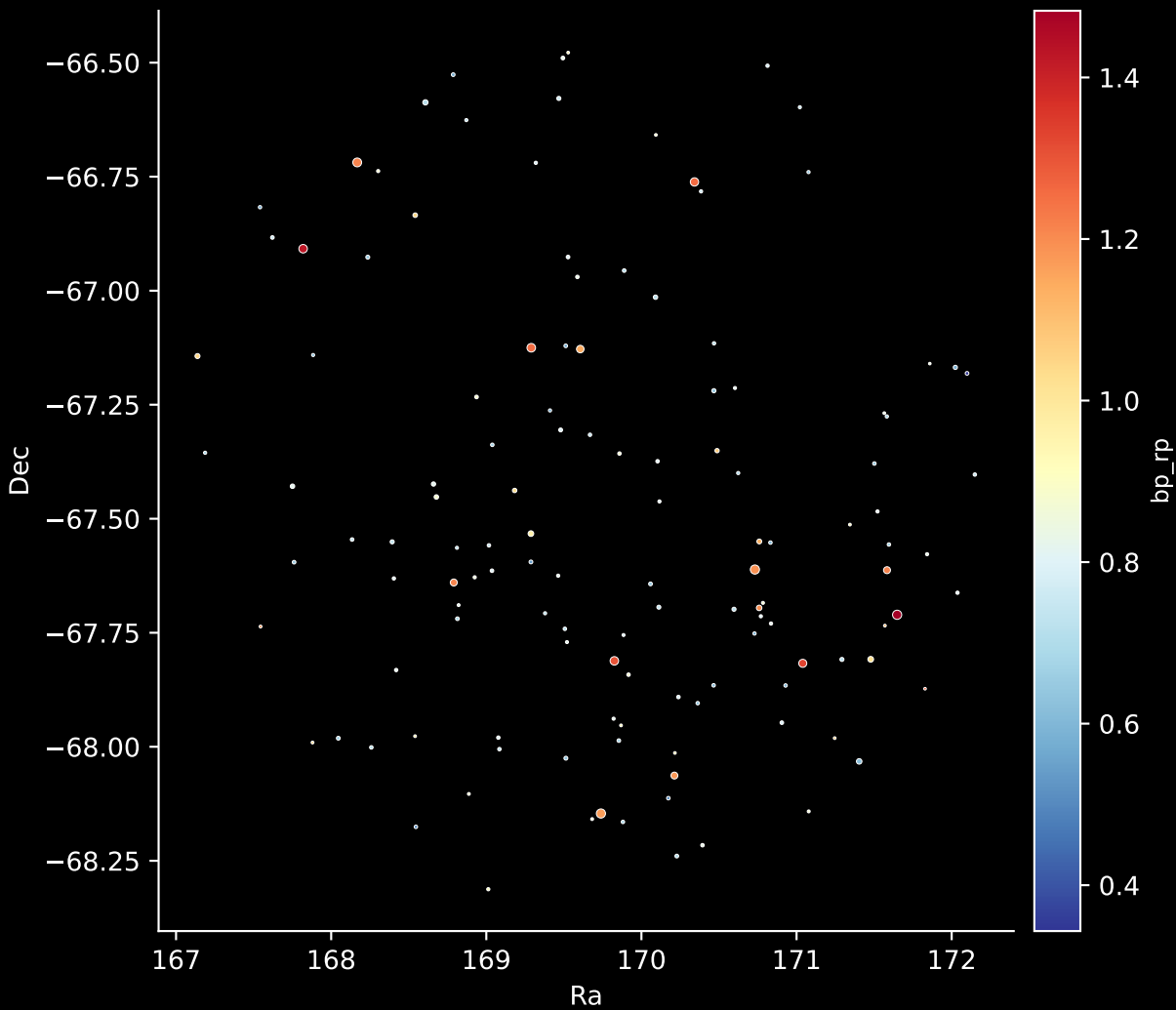
GALAH DR4 Field: [7178] Stars: 128
