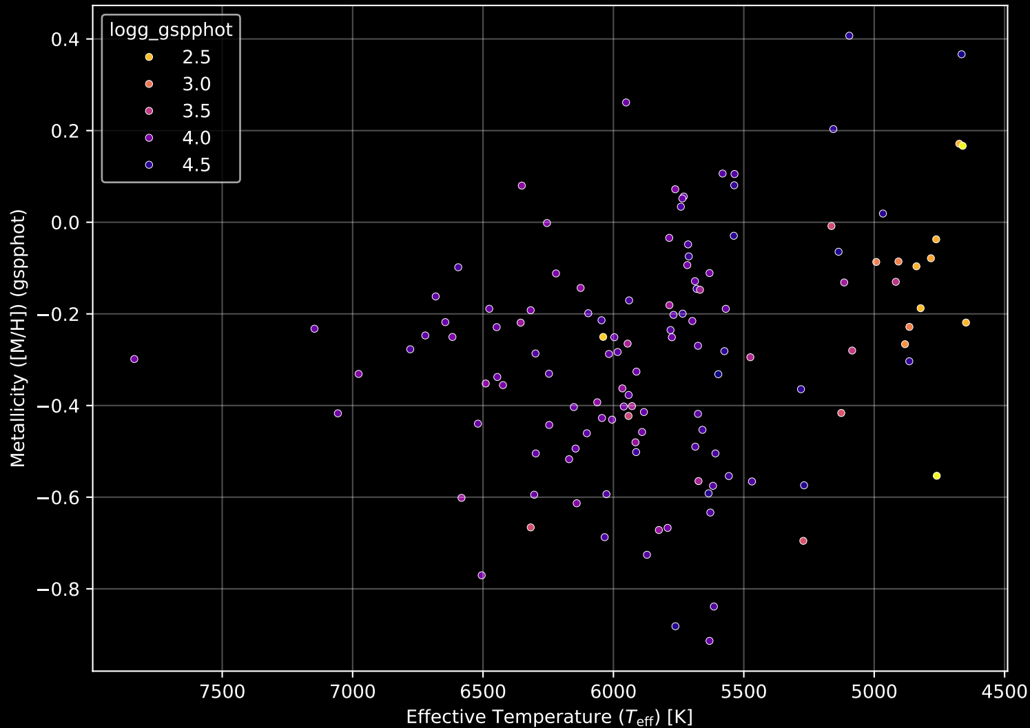
GALAH DR4 Field: [7178] Stellar Population Parameters (n= 128)
